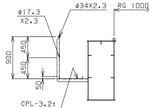
ガーダー断面
